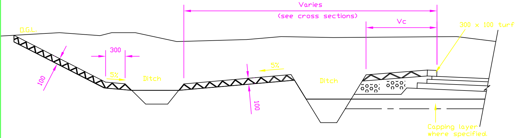
VERGE TYPE VG4(W)1
